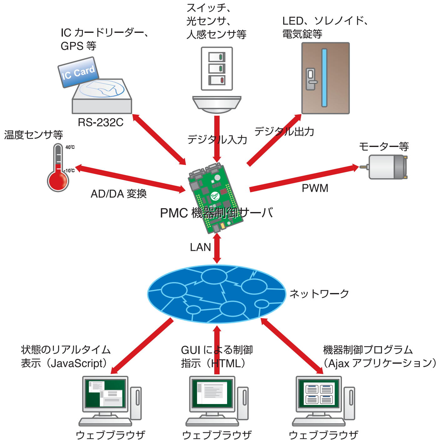
図 1. PMC 機器制御サーバの動作概念図
