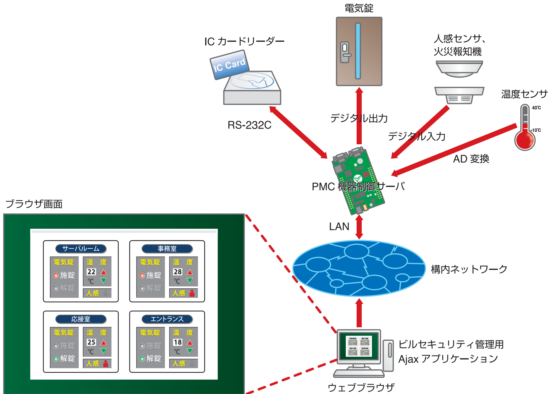
図 2. ビルセキュリティシステムへの応用例
