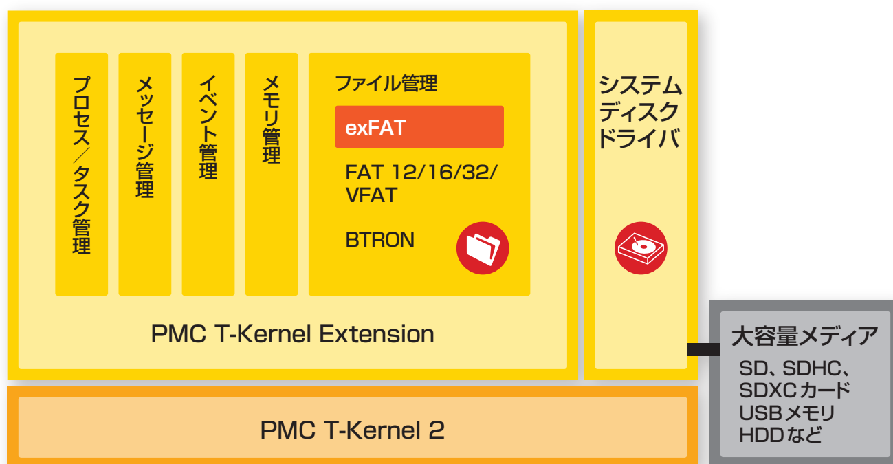
「exFAT for PMC T-Kernel」の構成図
