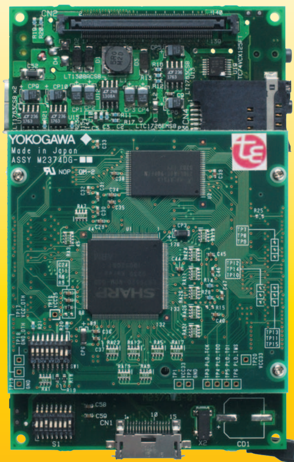
T-Engine/ARM720-LH7開発キットのCPUボード(原寸大)
