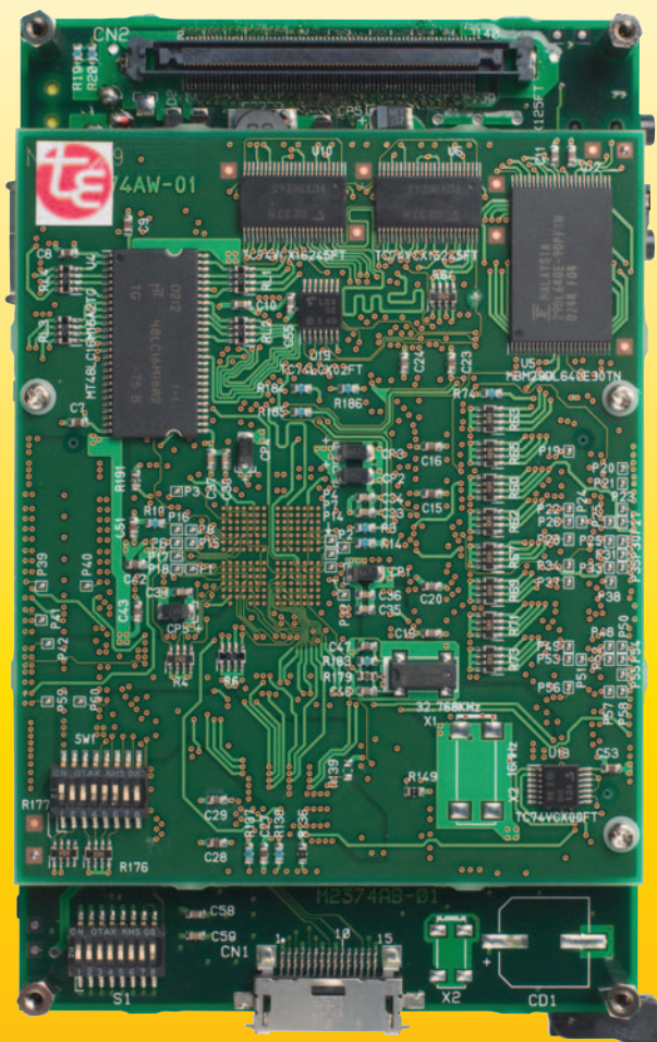
T-Engine/ARM920-MX1開発キットのCPUボード(原寸大)
