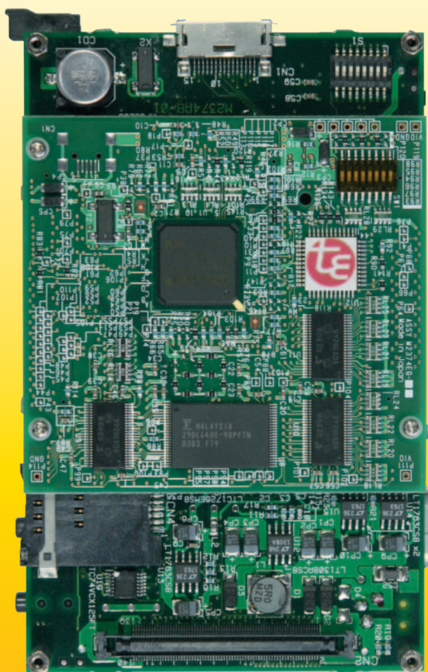
T-Engine/ARM922-LH7開発キットのCPUボード(原寸大)
