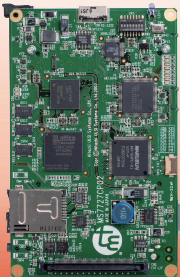
T-Engine/SH7727開発キットのCPUボード(原寸大)
